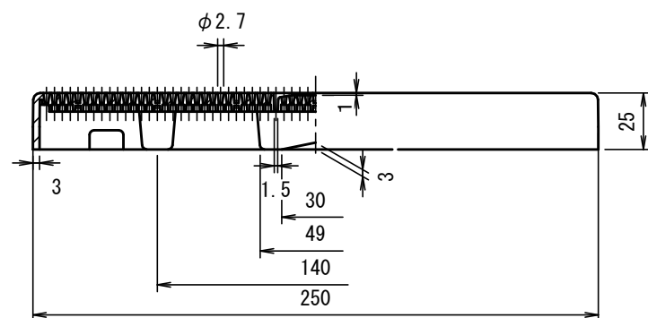
B-B断面図
