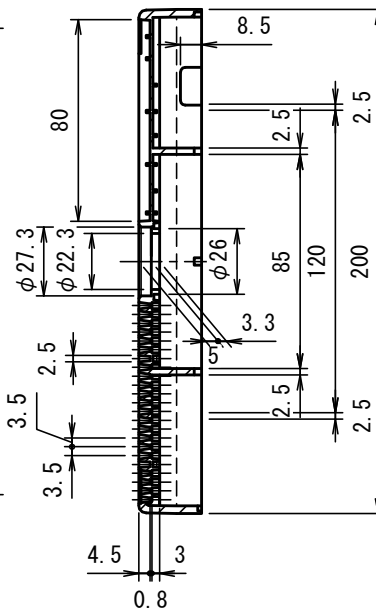
A-A断面図
